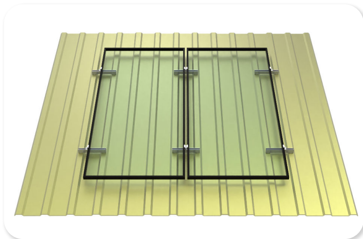
Montaje de greca a greca (30CM)
