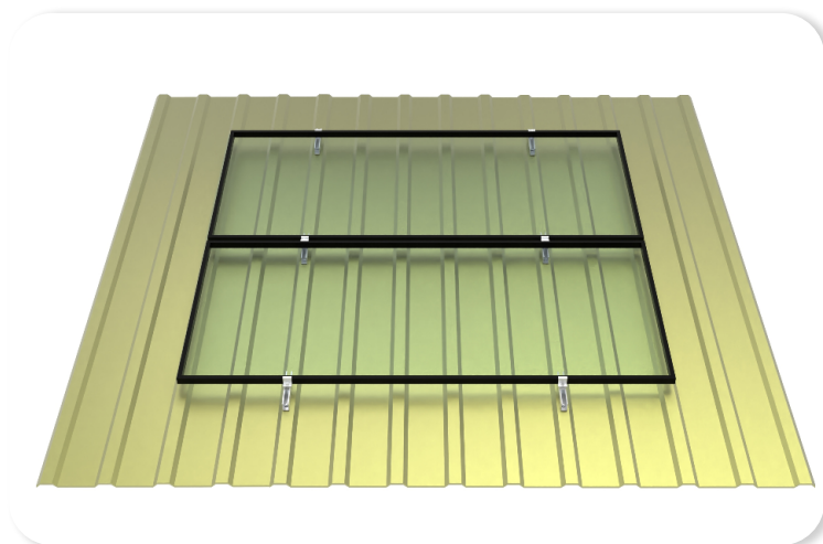
Montaje sobre greca (15CM)
